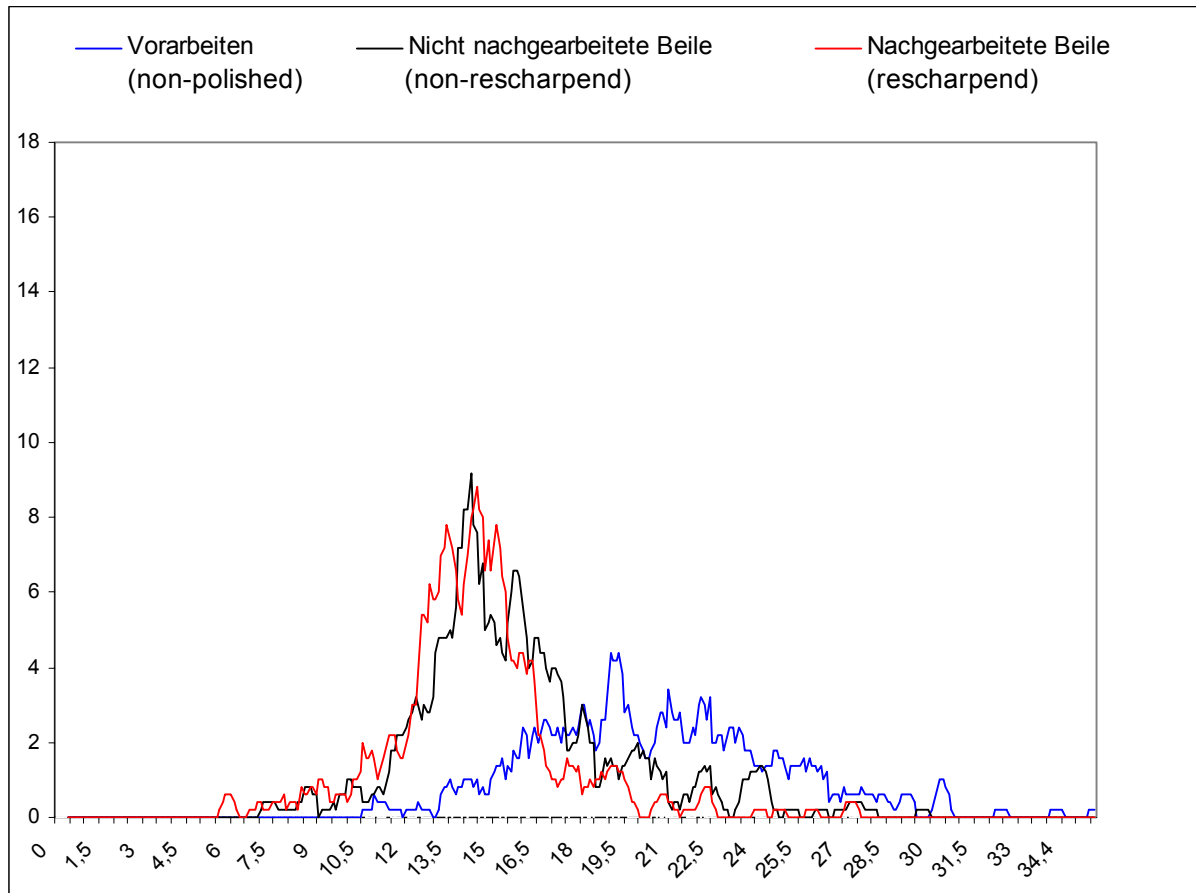
Diagr. 1: Längenvergleich von nicht nachgearbeiteten, nachgearbeiteten und ungeschliffenen dünnnackigen Flintbeile der Kreise Schleswig-Flensburg und Nordfriesland, Schleswig-Holstein.
