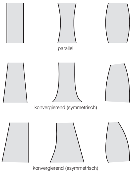
Abb. 17: SDS. Verlauf der Schmalseiten bei Flint- und Felssteinbeilen. Die Blickrichtung ist auf die Breitseite gerichtet.
